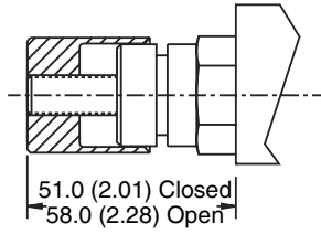
Knob Option
