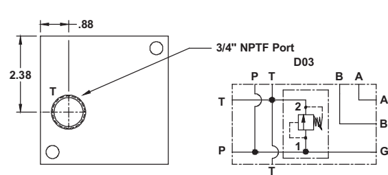
SPRP_03GSTSFUCA - BOTTOM VIEW
